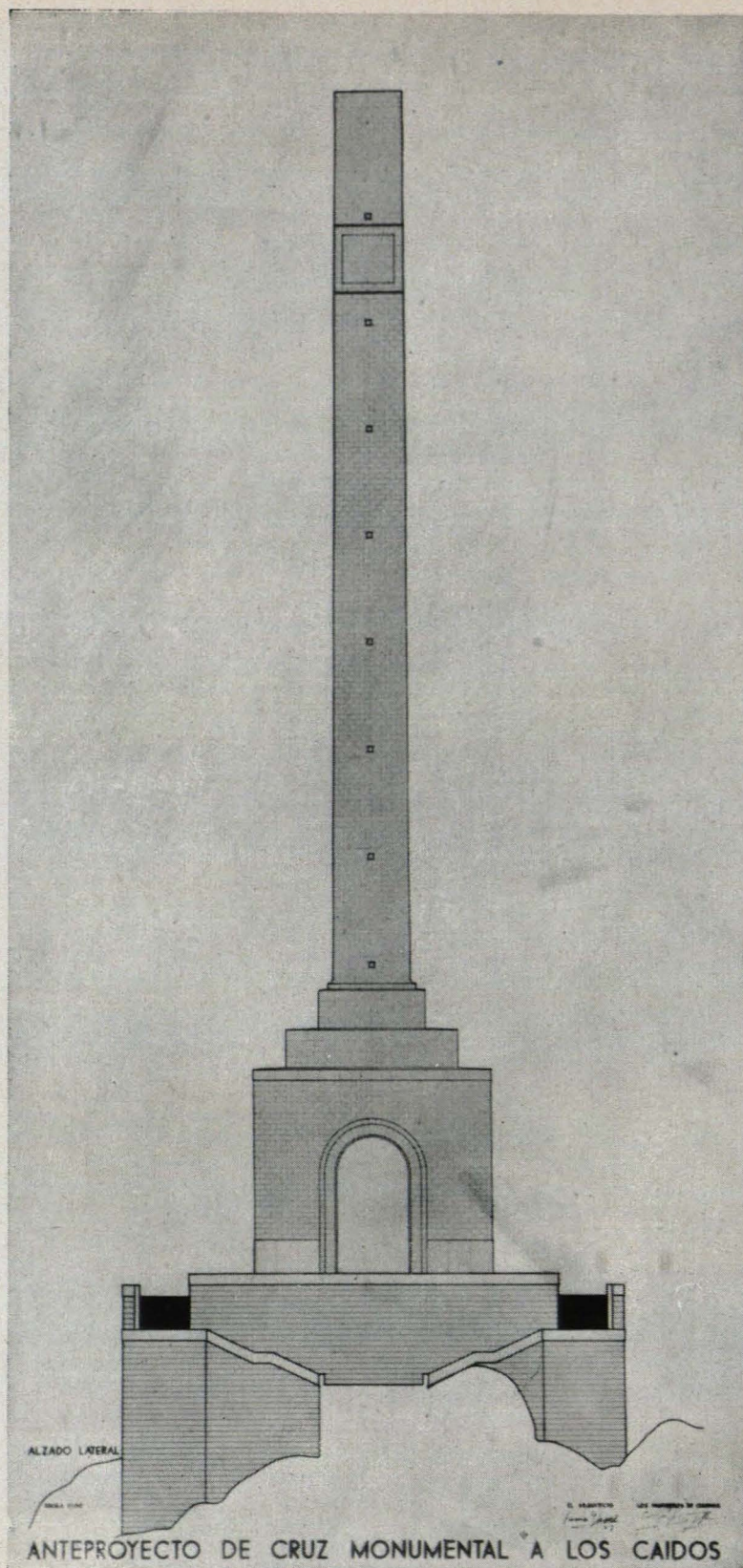
Alzado lateral
